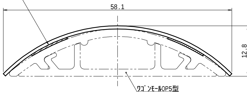
断面図 (2/1)
